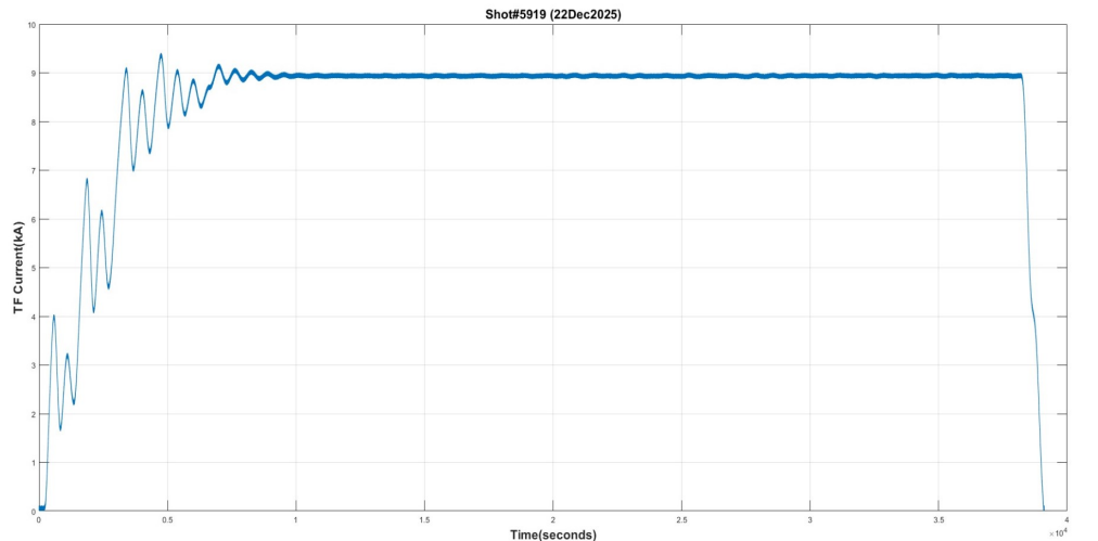
लगभग 9 kA करंट पर 9 घंटे तक टीएफ कॉयल की चार्जिंग दर्शाने वाला चित्र
