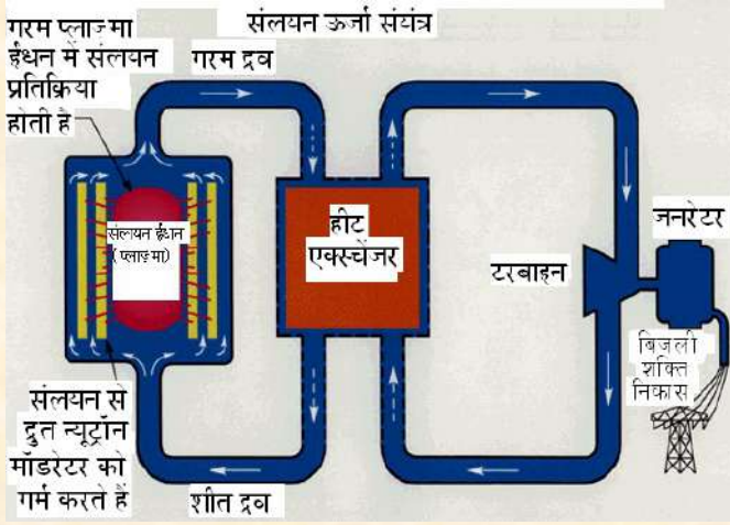
चित्र 3 : नाभिकीय संलयन रिएक्टर के घटक
